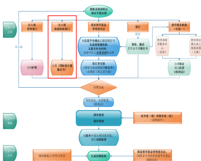
派出流程
